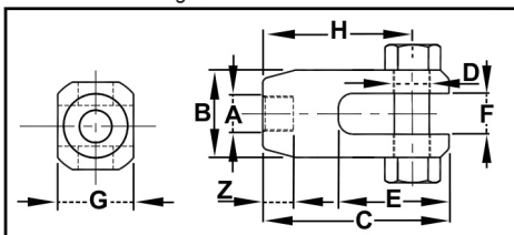
CPXX-Clevis Plunger & Base
